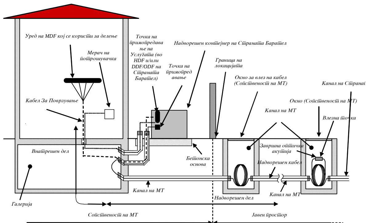
Слика 2 Шематски преглед на Оддалечена Колокација
